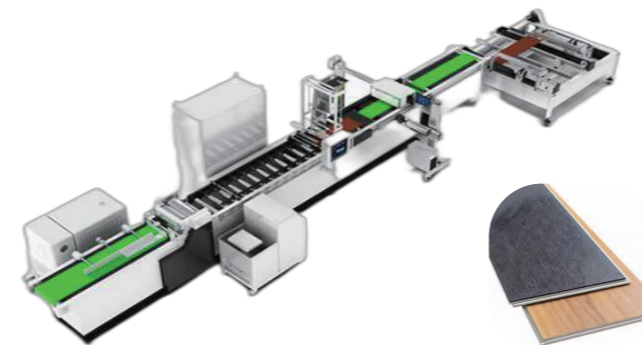
IXPE
